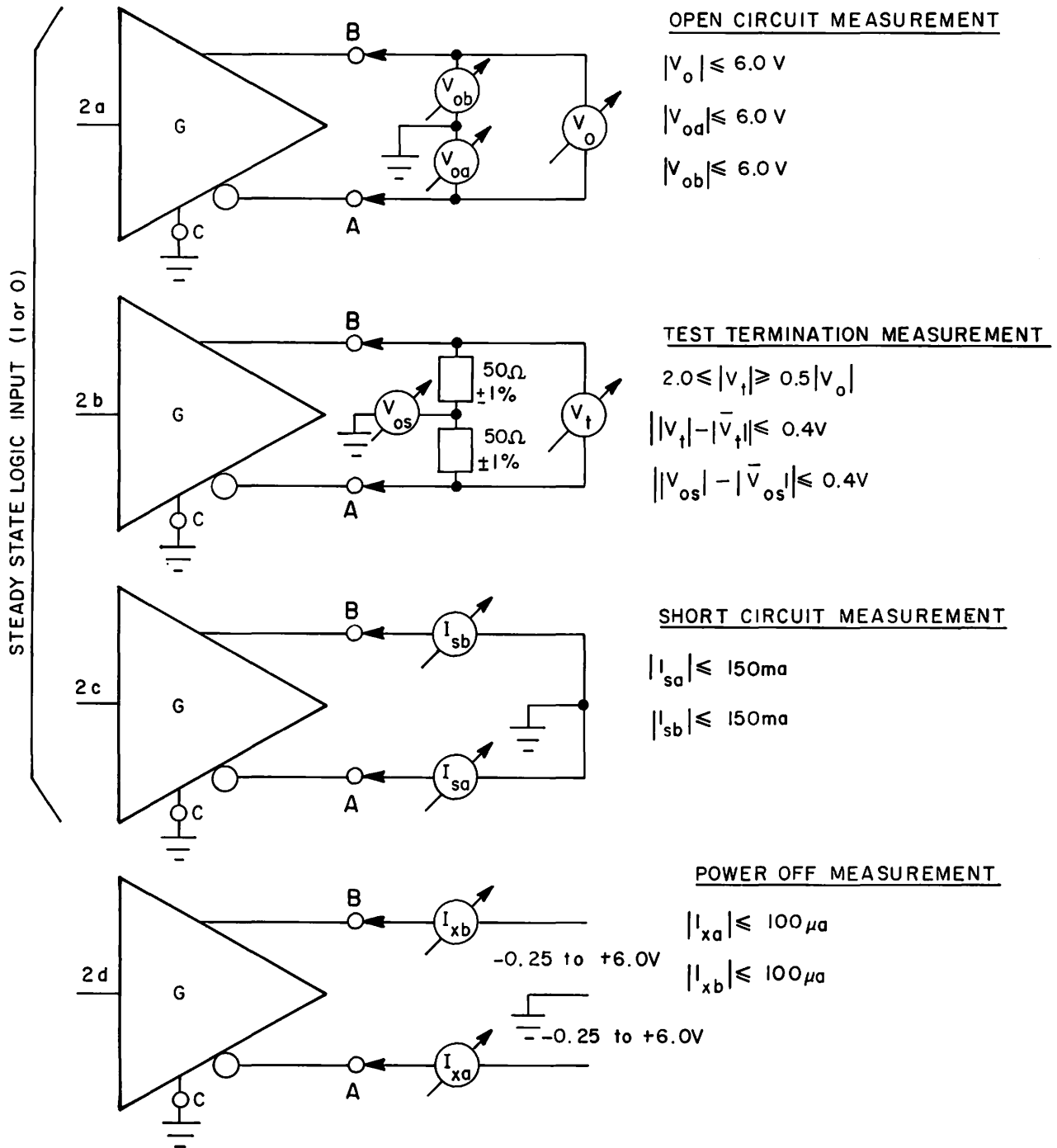
Fig. 2 Generator Parameter Measurement
