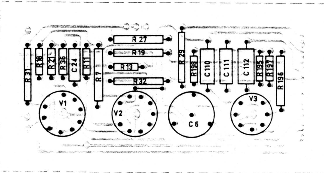
Input Amplifier
